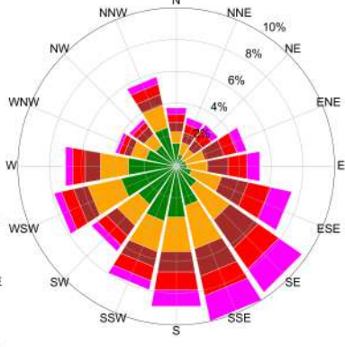
RVL 1 - eNose 10
